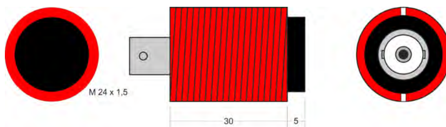
Fig. 4: Stator antenna A4b_PCM
